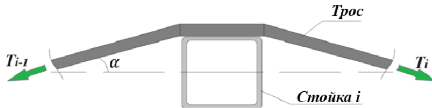
Рисунок 1 – Схема к определению падения усилия натяжения в тросе
