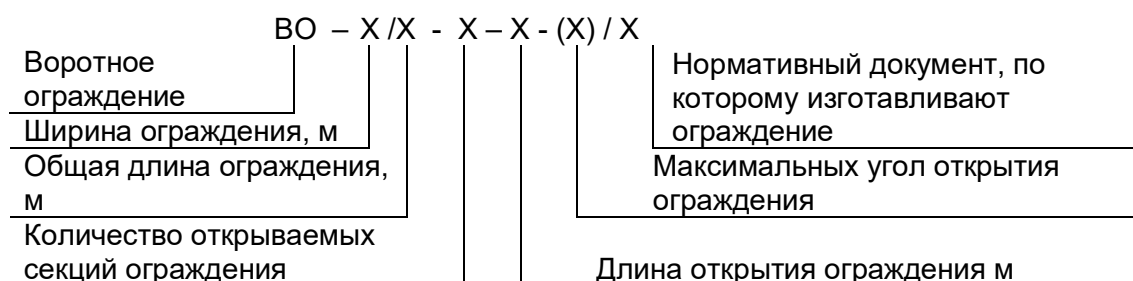
Рисунок А.1 — Последовательность расположения букв и цифр условного обозначения марки бокового ограждения воротного типа
